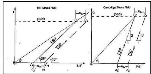
Figure 18 : MIT and Cambridge Stress Path Plot
